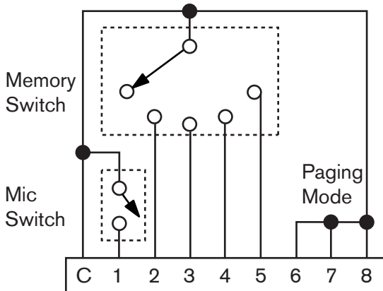
MRP Wiring
